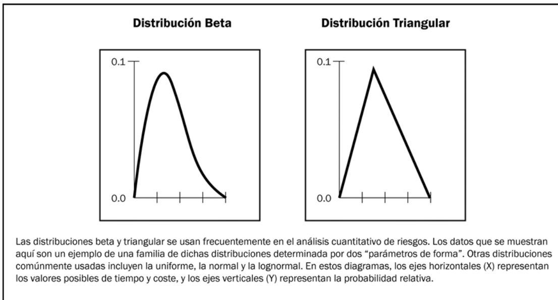
Figura 11-11. Ejemplos de Distribuciones de Probabilidad Comúnmente Usadas
